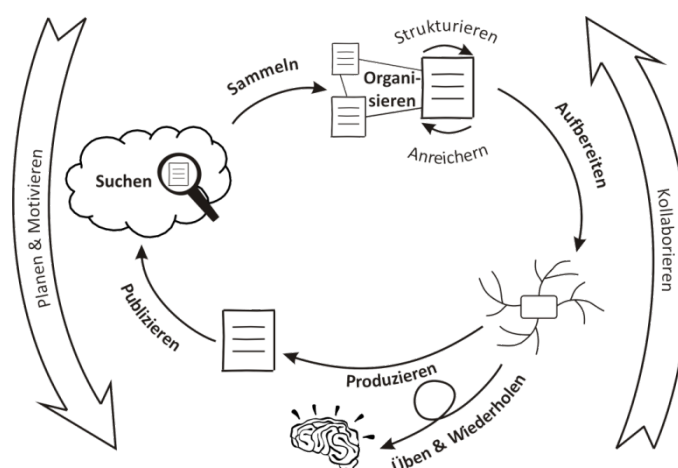
Abbildung 1: Idealisierter Lernprozess
